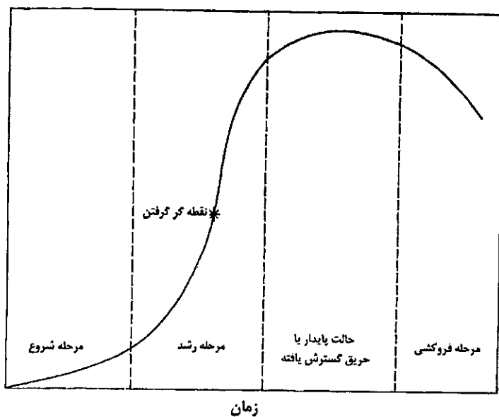
شکل پ-۲-۴: منحنی استاندارد رشد آتش‌سوزی
